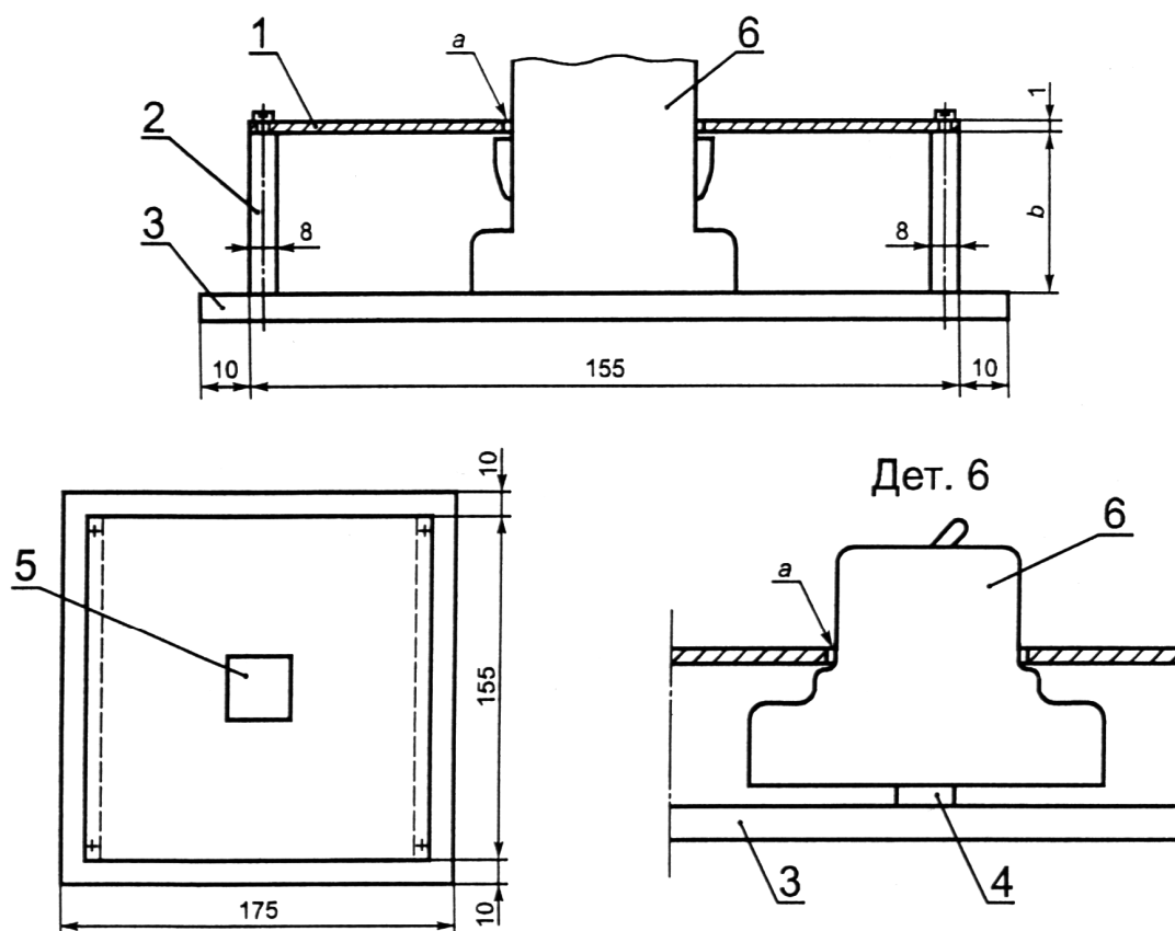
Рисунок 12 - Монтажная опора для испытаний на механический удар ( 9.13.2 )
