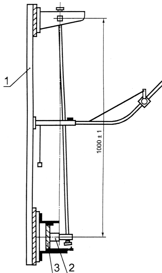
Рисунок 10 - Устройство для механических испытаний на удар
