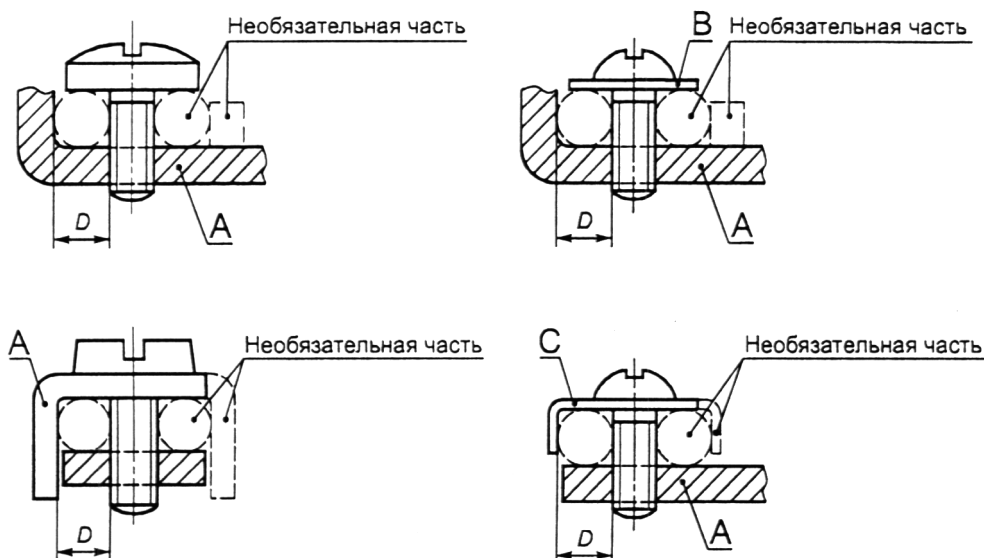
Рисунок F. 1 - Примеры столбчатых выводов
