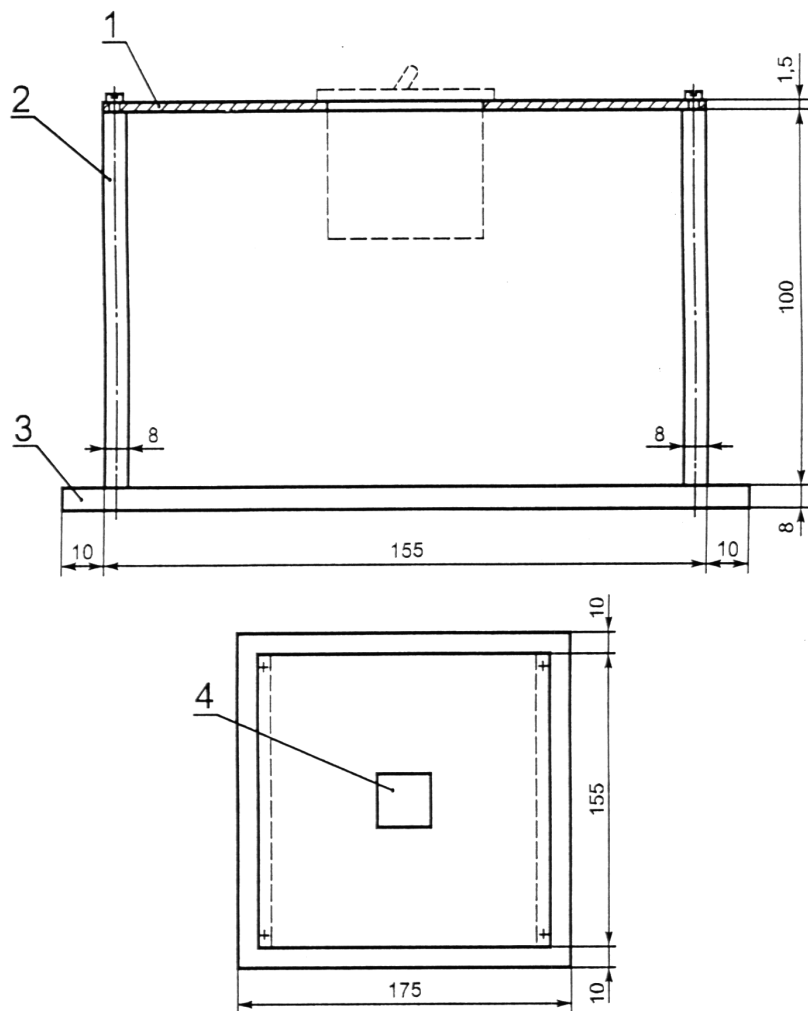
Рисунок 13 - Пример монтажа автоматического выключателя утопленного монтажа для испытаний на механический удар
