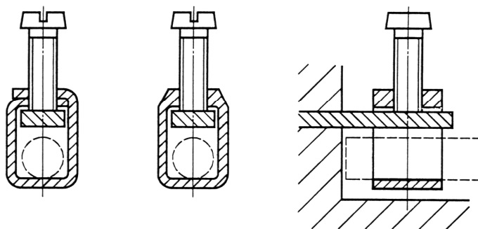
Выводы с хомутиком
