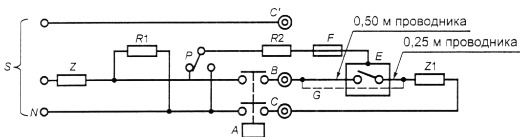
Рисунок 3 - Однополюсный автоматический выключатель
