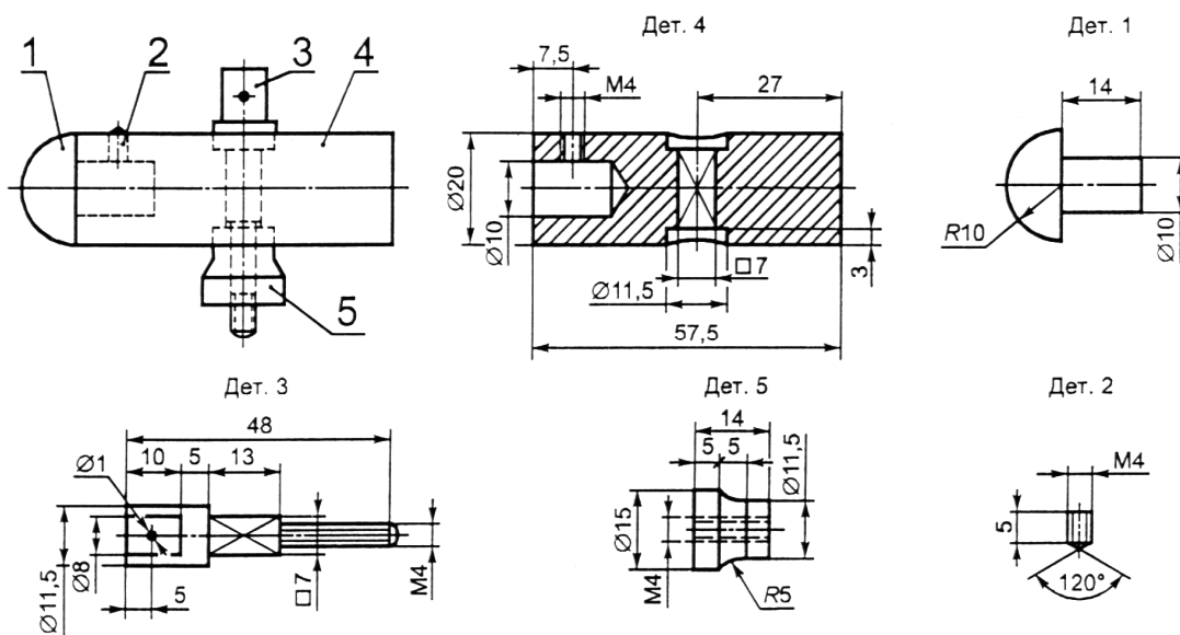
Рисунок 10 - Устройство для механических испытаний на удар
