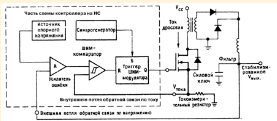
Рис. 2. При регулировании с использованием ШИМ-модуляции и дополнительной обратной связи по току дросселя (ДОСТА) ключ выключается при достижении током дросселя некоторого порогового значения. Порог задается выходным сигналом усилителя ошибки и величиной напряжения на токоизмерительном резисторе
