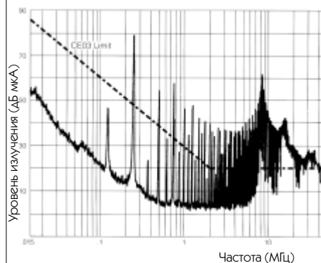
Рис. 1а. Уровень помех на входе преобразователя MHE 2805S без дополнительного фильтра
