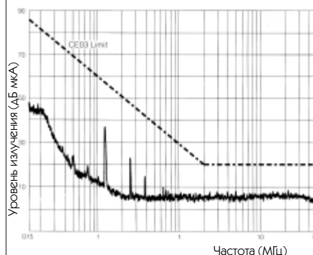
Рис. 1б. Уровень помех на входе преобразователя MHE 2805S с фильтром FMH-461
