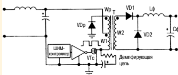
Рис. 1а. Преобразователь с размагничивающей обмоткой
