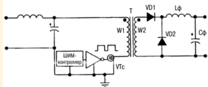
Рис. 1б. Преобразователь с АРТ
