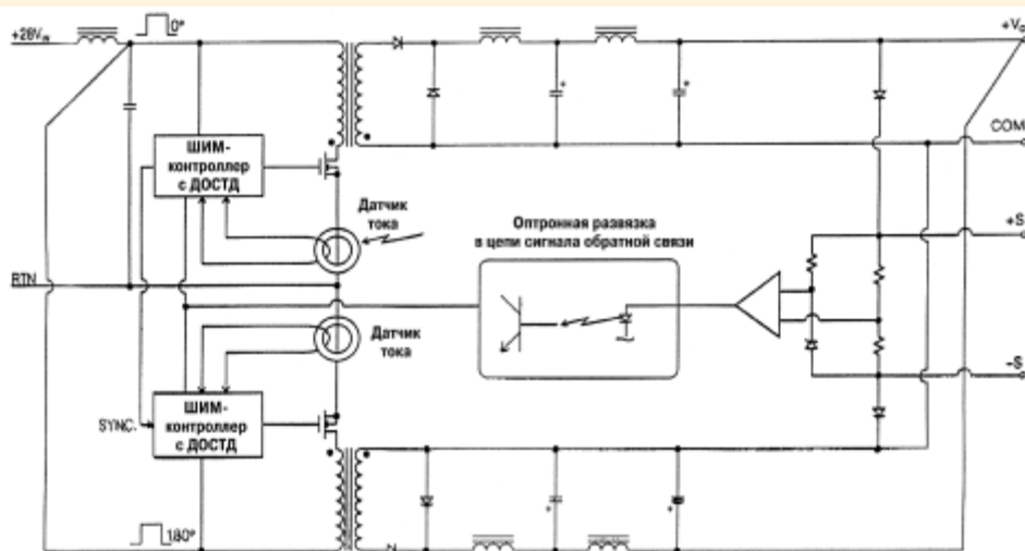
Рис. 3. Функциональная схема преобразователя МК200
